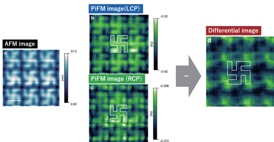
図4 光誘起力顕微鏡による近接場CDイメージング [5] 。(a)トポグラフィ像、(b,c)左右円偏光励起による光誘起力像、(d)それらの差分像（CDに対応）。CC-BY-NC-ND 4.0 © 2023 American Chemical Society.
