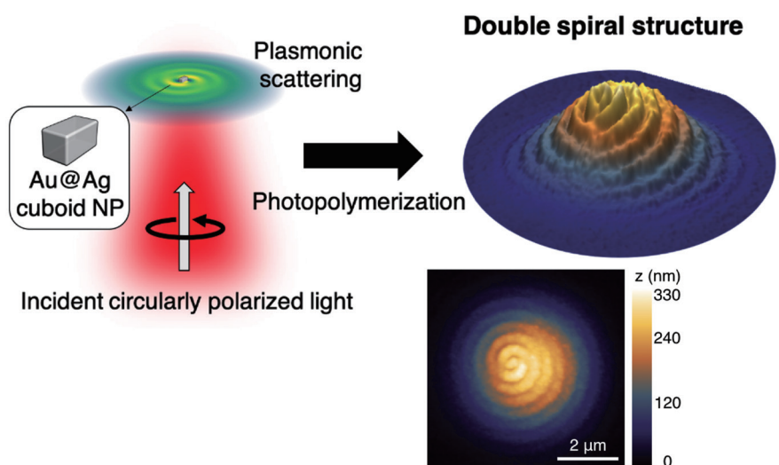
図6 金属直方体ナノ微粒子の円偏光照射に伴う光重合反応で生成した渦状ナノ・マイクロ構造体 [14] 。CC-BY-NC-ND 4.0 © 2024 American Chemical Society.
