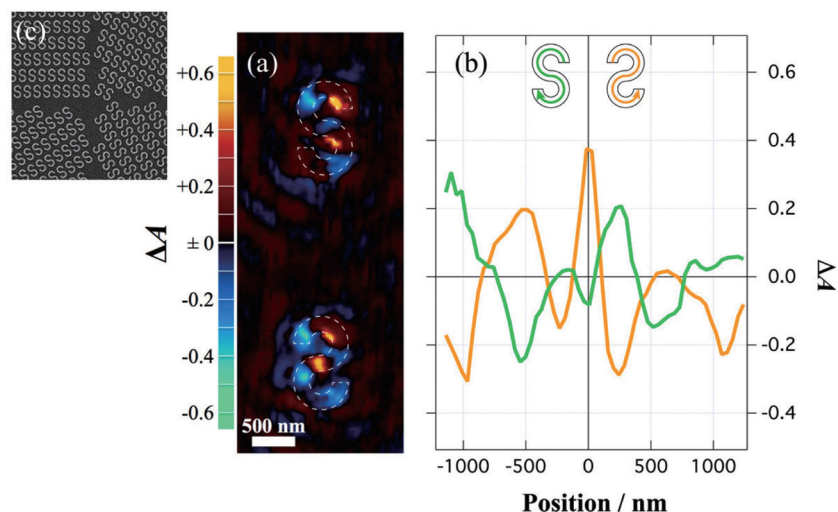
図2 (a)S字型とその鏡像体の金ナノ構造の近接場CDイメージング、(b)S字曲線に沿ったCD信号のラインプロファイル、(c)試料の走査電子顕微鏡写真 [1] . Reproduced with permission © 2013 American Chemical Society.
