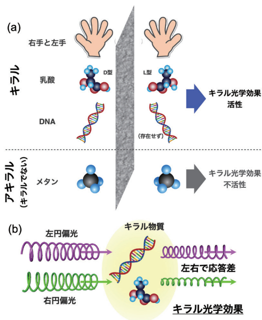
図1 (a)キラルとアキラル(キラルでない)な構造と、キラル光学効果の活性・不活性。(b)キラル光学効果の一つとしての、円偏光二色性。キラル物質は、左円偏光と右円偏光に対する光吸収の大きさが異なる。
