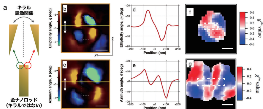
図3 (a)キラルでない金ナノロッドについて、左上と右上は、局所的にはキラルな構造で、互いに鏡像関係にある。(b-e)金ナノロッドの近接場ポラリメトリ [3] 。(b)楕円率像 (CDに対応)、(c)偏光回転角像 (ORに対応)、(d,e)それぞれの図中の黄線に沿ったラインプロファイル。Reproduced with permission © 2018 American Chemical Society. (f)短い金ナノロッド、(g)長い金ナノロッドの近接場二光子励起CD像 [4] 。(f)は(b)と同様のモード、(g)は高次のモードによるキラル光学効果。Reproduced with permission © 2016 American Chemical Society.
