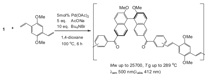
図3 Pdナノクラスター触媒を用いる溝呂木-Heckカップリング重合による溶剤可溶性ポリアリーレンビニレンケトン (PAVK) の合成
